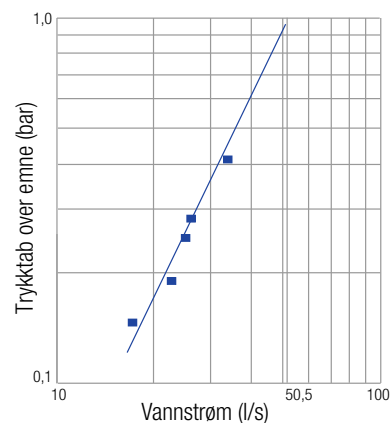
Flowtest for brannpost serie 09 Flowtest utført på en DN100 brannpost med totallengde på 1900 mm Kv = 180
